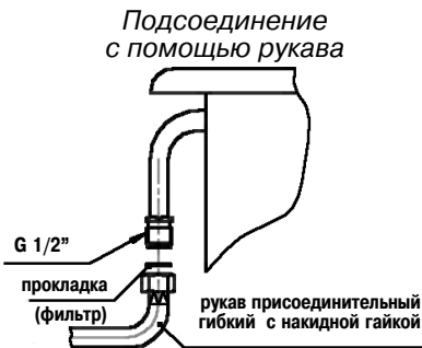
Рис.3 Подсоединение гибким газовым шлангом с накидной гайкой
