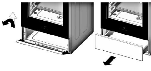
Дверь нижняя Ящик Рис. 11 Открывание хозяйственного отделения
