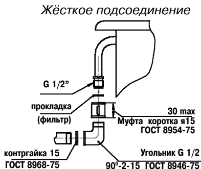
Рис.4 Жесткое подсоединение
