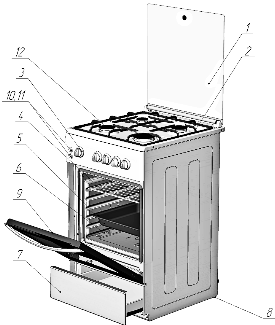
Рис. 7 Устройство плиты
