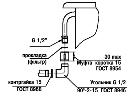
Мал.4 Жорстке приєднання.
