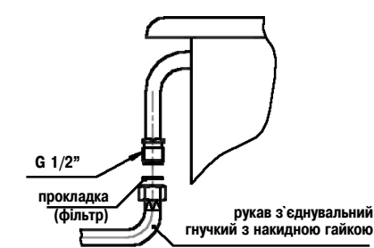
Мал.3 Приєднання гнучким газом шлангом з накидною гайкою.
