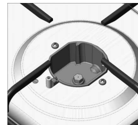
Рис. 5 Сопло S7 в корпусе сопла
