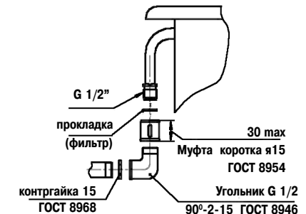
Рис.4 Жесткое подсоединение
