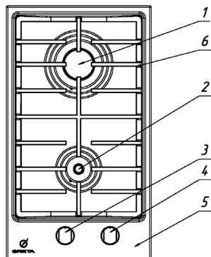
мал. 5 Устрій столу вбудованого
